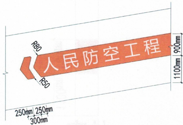
图2 非机动车坡道侧墙标识样式示例
