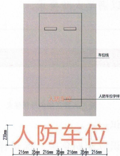
图5 人防车位标识喷绘样式
